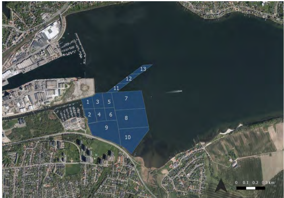
Figur 4-1: Oversigtskort over området for uddybning til Marina City. Uddybningsområdet er markeret med blå rektangler.
