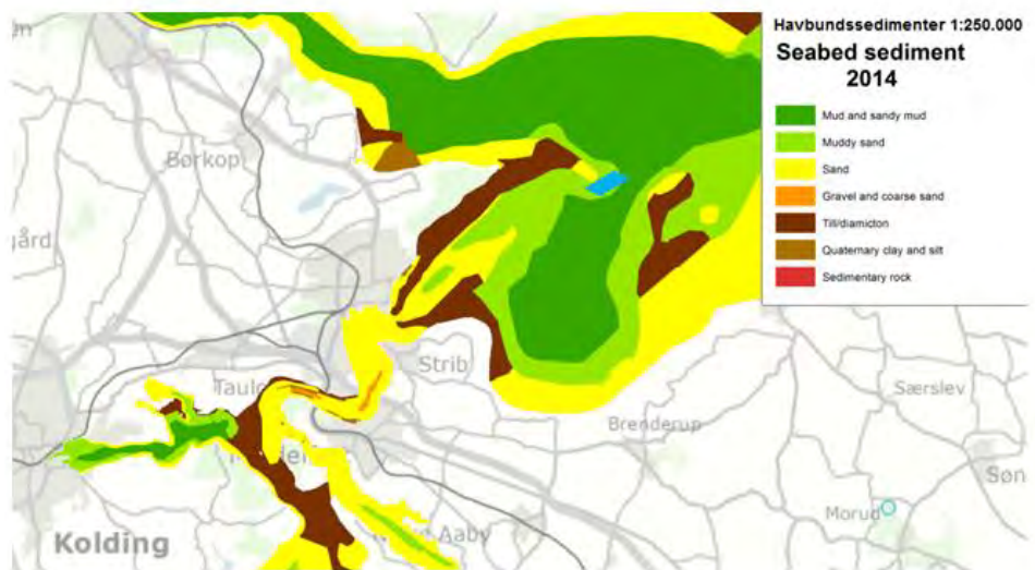
Figur 5-2 Kort over sedimenttyper i Kolding Fjord og ved klapplassen Trelde Næs. Omtrentlig placering af klapplassen er angivet med blå firkant. Data fra (GEUS, 2017).
