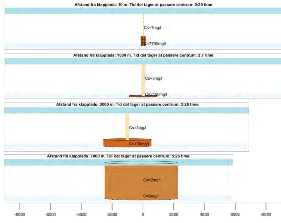
Figur 7-6: Sedimentpølen udbredelse i vandsøjlen samt på tværs af sundet ud for Vejle Fjords udmundning i de samme afstande fra klappositionen som i Figur 7-5. I figuren er det også angivet, hvor lang tid det tager for sedimentpølen at passere centrum.
