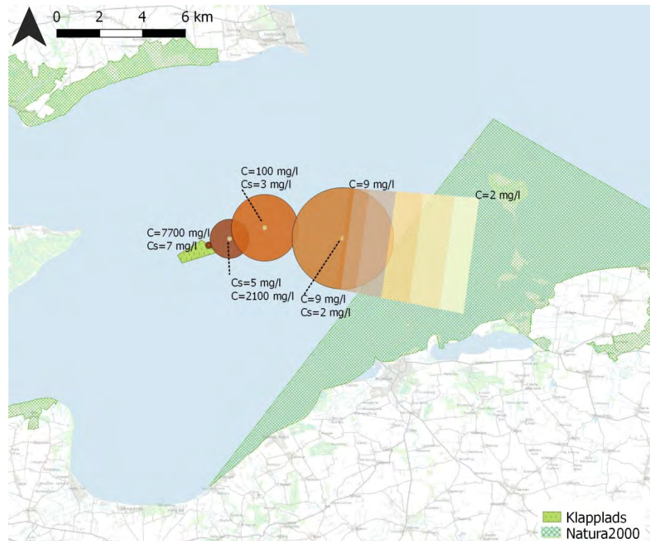
Figur 7.3: Spredning af sedimentpøl i nordlig retning. Figuren viser sedimentpølenes placering, størrelse og koncentration, C , henholdsvis 10, 1000, 3000 og 7000 m fra klappositionen, samt hvordan sedimentet vil spredes, når sedimentpølen opløses 7.000 m fra klappositionen. Sedimentkoncentrationen af de 5 % sediment tabt i vandsøjlen i midten af sedimentpølen, C_s , til samme tid er også angivet i figuren. Værdierne af disse er aflæst i MIKE-beregningerne.
