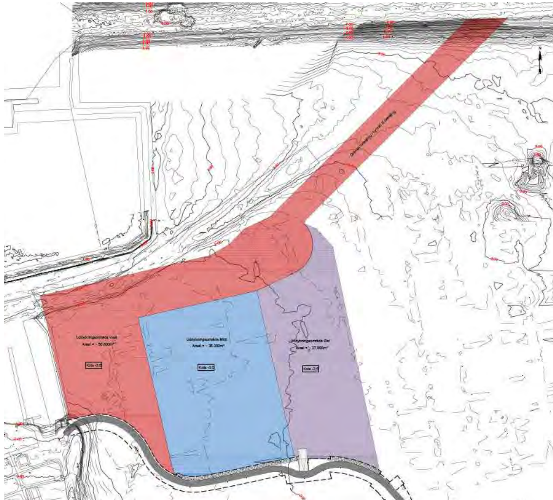
Skitse 3. Uddybning i marina og sejlrende
